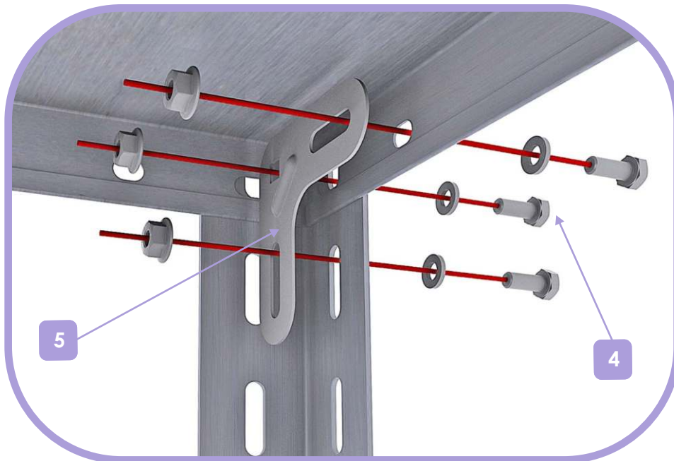
Detalle del atornillado de la escuadra a la balda y al ángulo.
